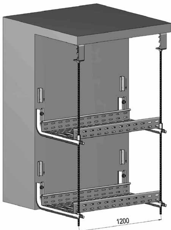
Oldalfali rögzítés, kiegészítő menetes szás biztosítással mennyezetre
