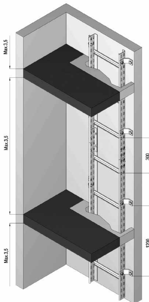
Felszálló nyomvonal, oldalfalhoz rögzítve
